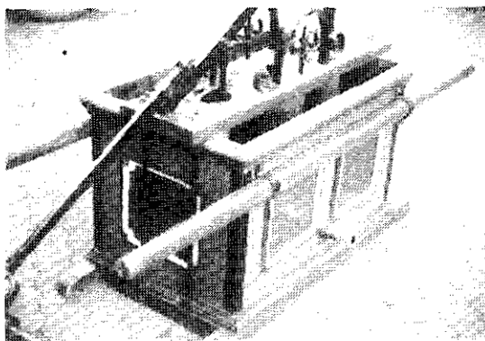
afb.3: draagbare brandspuit (midden 19de eeuw) van Rossdorg, het buurdorp van Mardorf, waar Heinrich Josef van Moll werkzaam was, zodat hij zo goed als zeker de maker van het toestel was.
